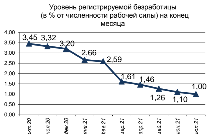
Диаграмма 2
